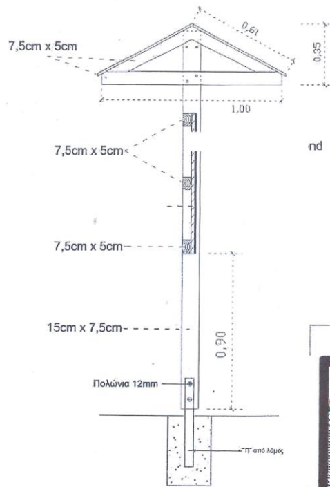
Πλάγια όψη
