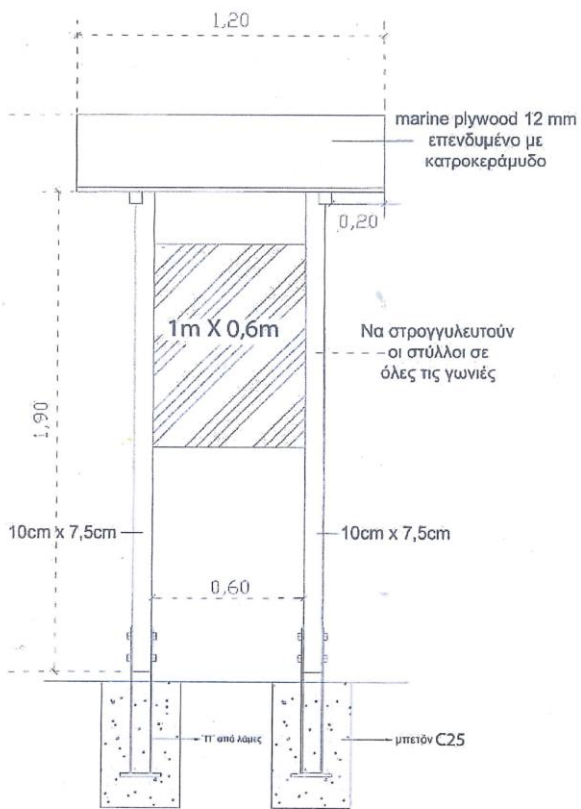
Πρόσοψη
